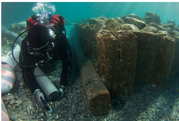
Fig. 4. Ioannis Sapountzis udgraver den nordlige side af Sænkekasse 5. I forgrunden til højre ses den vestlige side (Foto: V. Tsiiris 2015)
