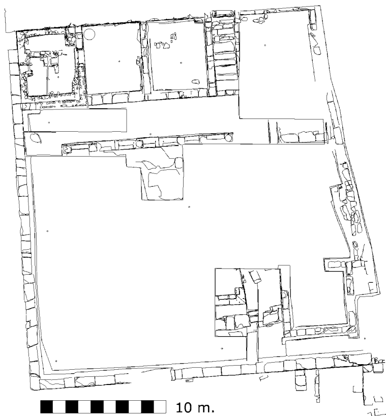
Plan over peristyl-bygningen efter udgravningerne i 2005. Indgangen er via trappen i den nordlige del, mens kultrummet ligger i det nordvestlige hjørne. På stylobatet mod nord ses ligeledes de otte søjlebaser.
