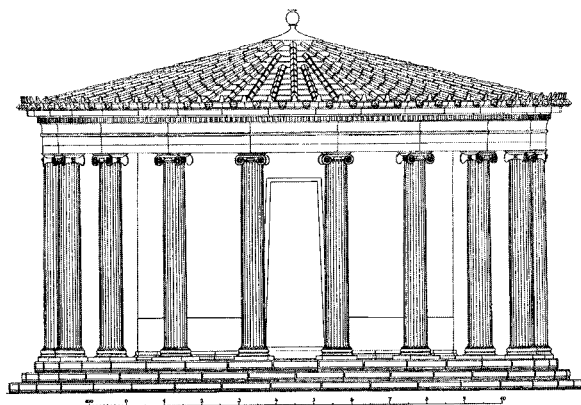
Fig. 17. Klaus Herrmanns seneste rekonstruktion af Philippeion i Olympia.
