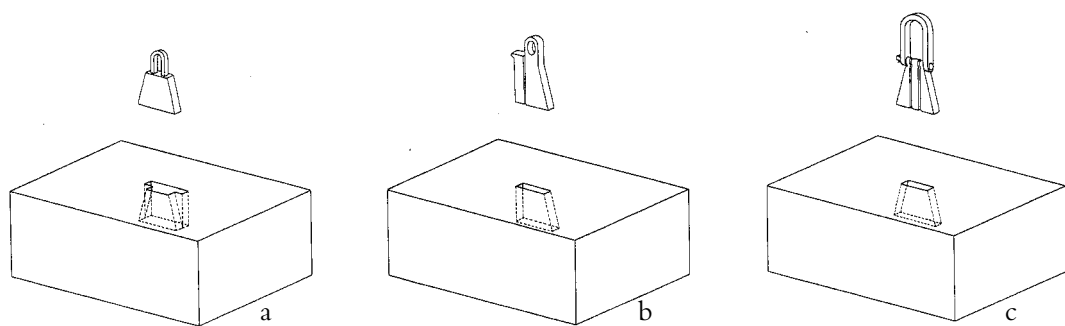
Fig. 4. Løftehuller i græsk-romersk arkitektur. Over hver er skitseret rekonstruktion af de tilhørende jernankre, hvortil en kæde eller tovværk var fastgjort. Til venstre ses det særlige østgræske løftehul fra Den ioniske Renæssance, anvendt formentlig ca. 370-150 f.Kr. I midten en tidlig udgave af det almindelige græsk-romerske løftehul, som ses til højre i den meget udbredte udgave, som er blevet anvendt gennem århundreder i antik og senere arkitektur.
