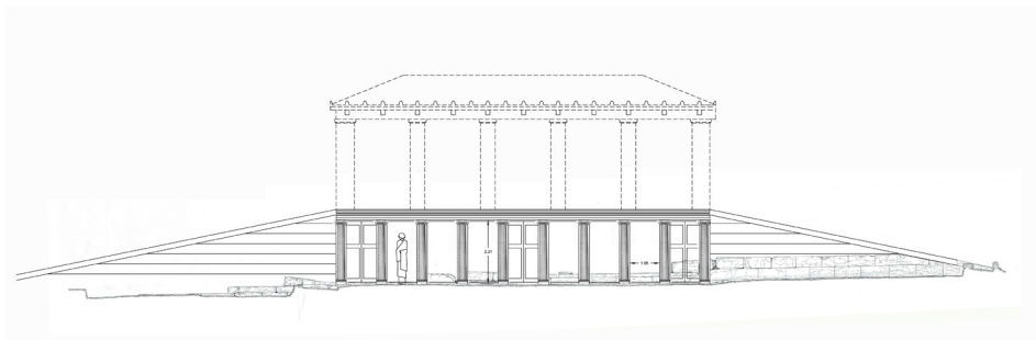
Fig. 4. Kalydons teater. Rekonstruktionstegning af scenebygningens front 2014 (N. Hatzidakis)
