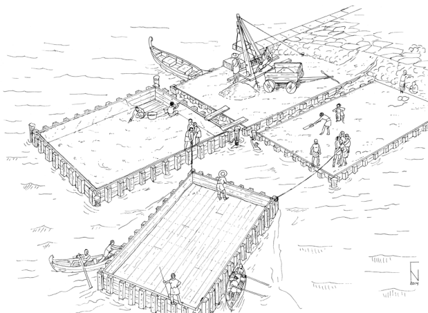
Fig. 8. Kunstnerisk rekonstruktion af sænkekasserne i område 2 (Y. Nakas 2014)
