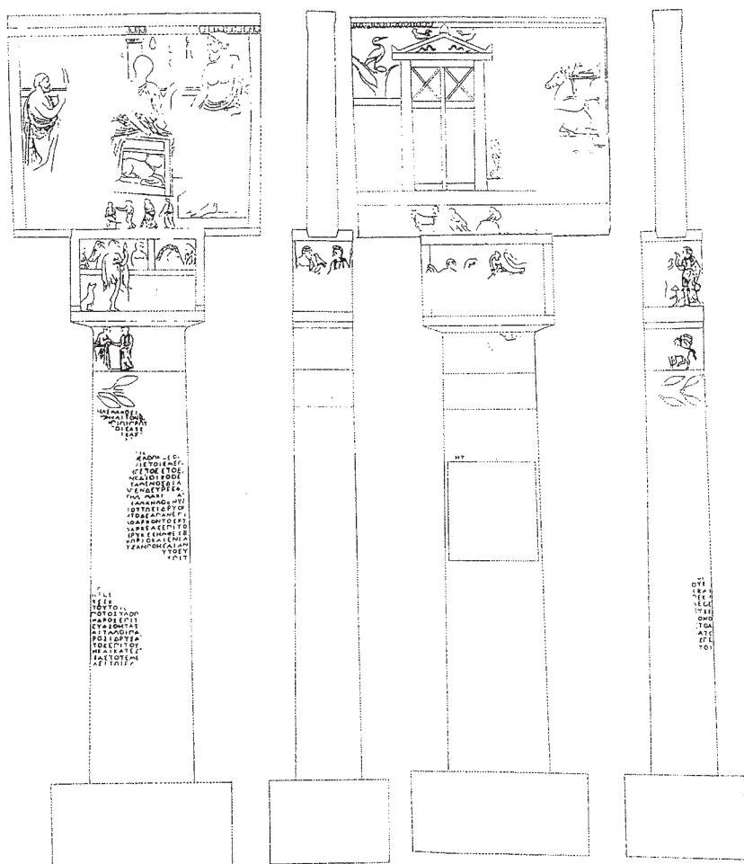
Tegning af Telemachos-monumentet efter L. Beschi 2002, ASAtene 80, 23, fig. 7.
