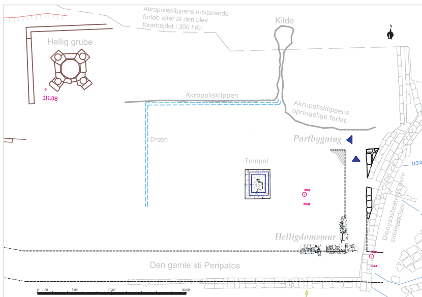
Grundplan af Asklepios-helligdommen fra 420-350 f.kr.
