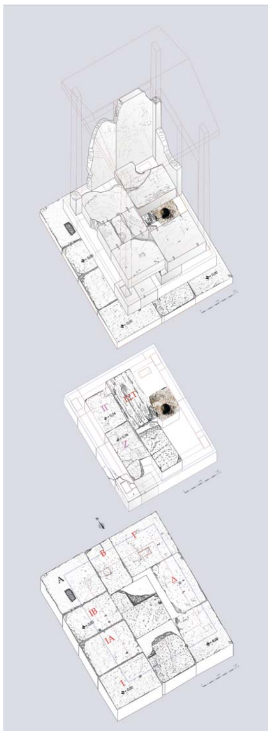
Rekonstruktion af templet i konstruktionsfase III med fundamentet, 1. trin og 2. trin med overbygningen.
