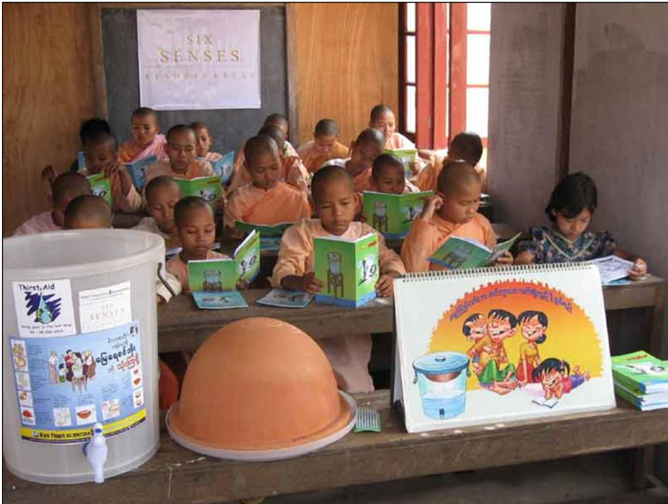
Filtros de cerámica tipo olla en Myanmar (Fuente: ThirstAid)
