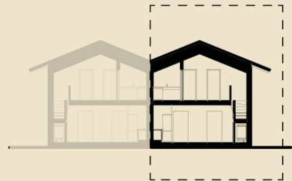
Snitt
