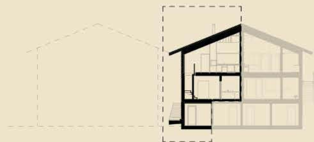
Snitt
