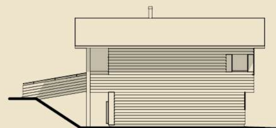
Fasade øst
