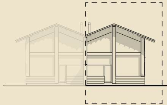
Fasade nordvest
